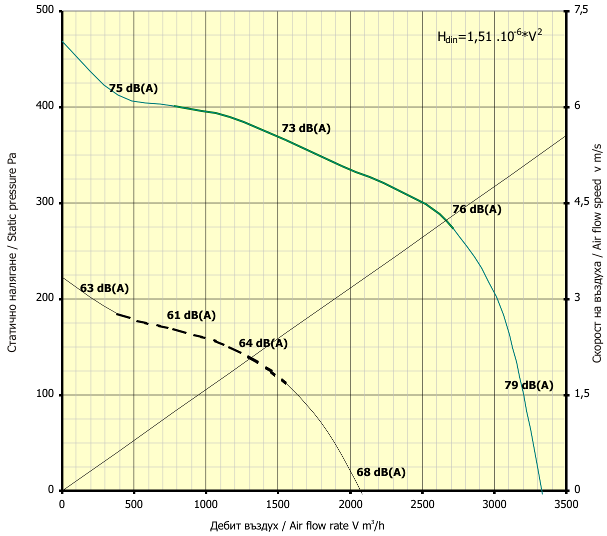
Характеристики на центробежен вентилатор Characteristics of centrifugal fans range KVB-240-500/350 A1
