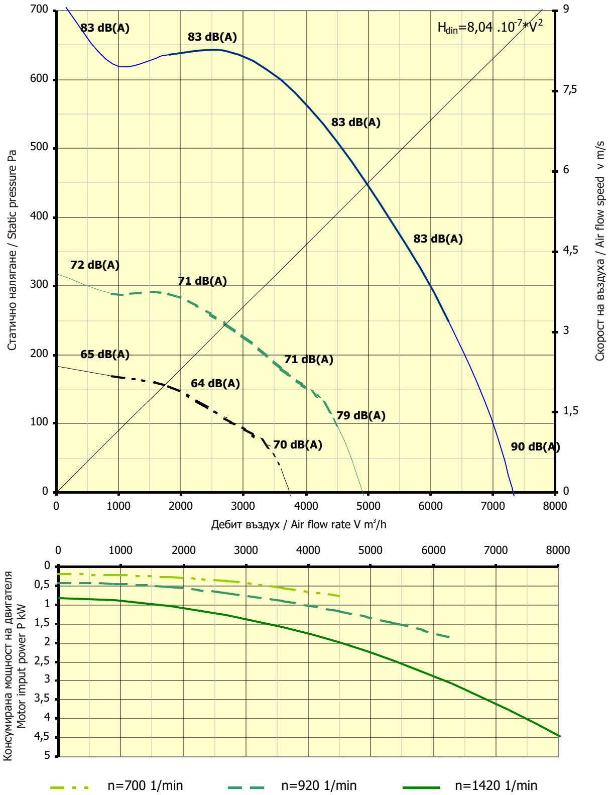
Характеристики на центробежен вентилатор Characteristics of centrifugal fans range KVB-315-600/400 A3
