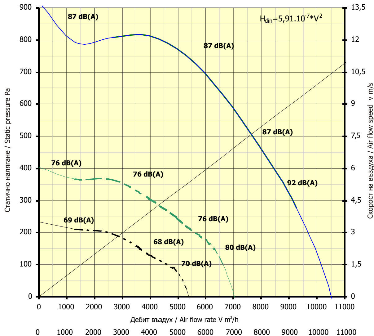
Характеристики на центробежен вентилатор Characteristics of centrifugal fans range KVB-355-700/400 A3
