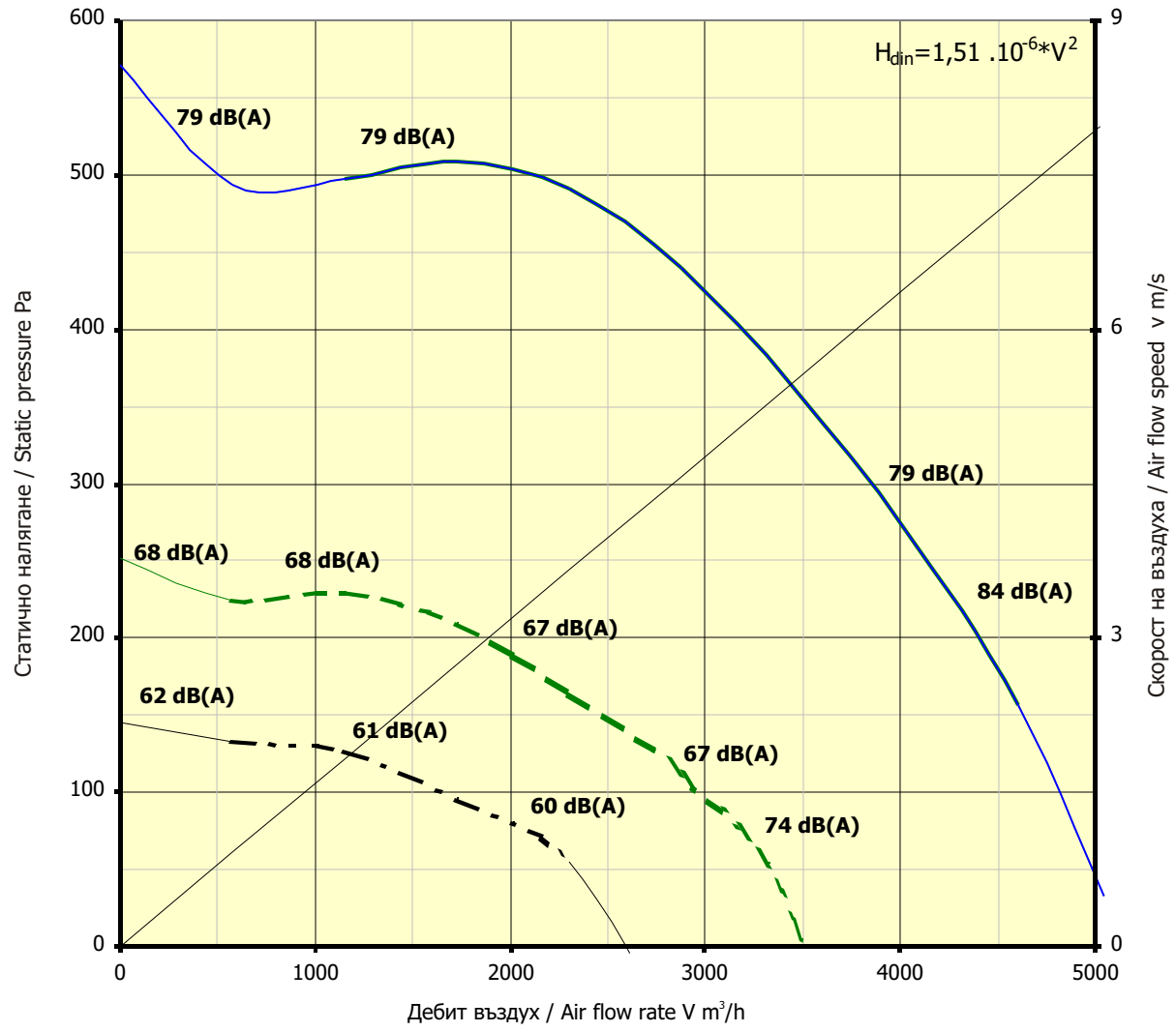
Характеристики на центробежен вентилатор Characteristics of centrifugal fans range KVB-280-500/350 A3
