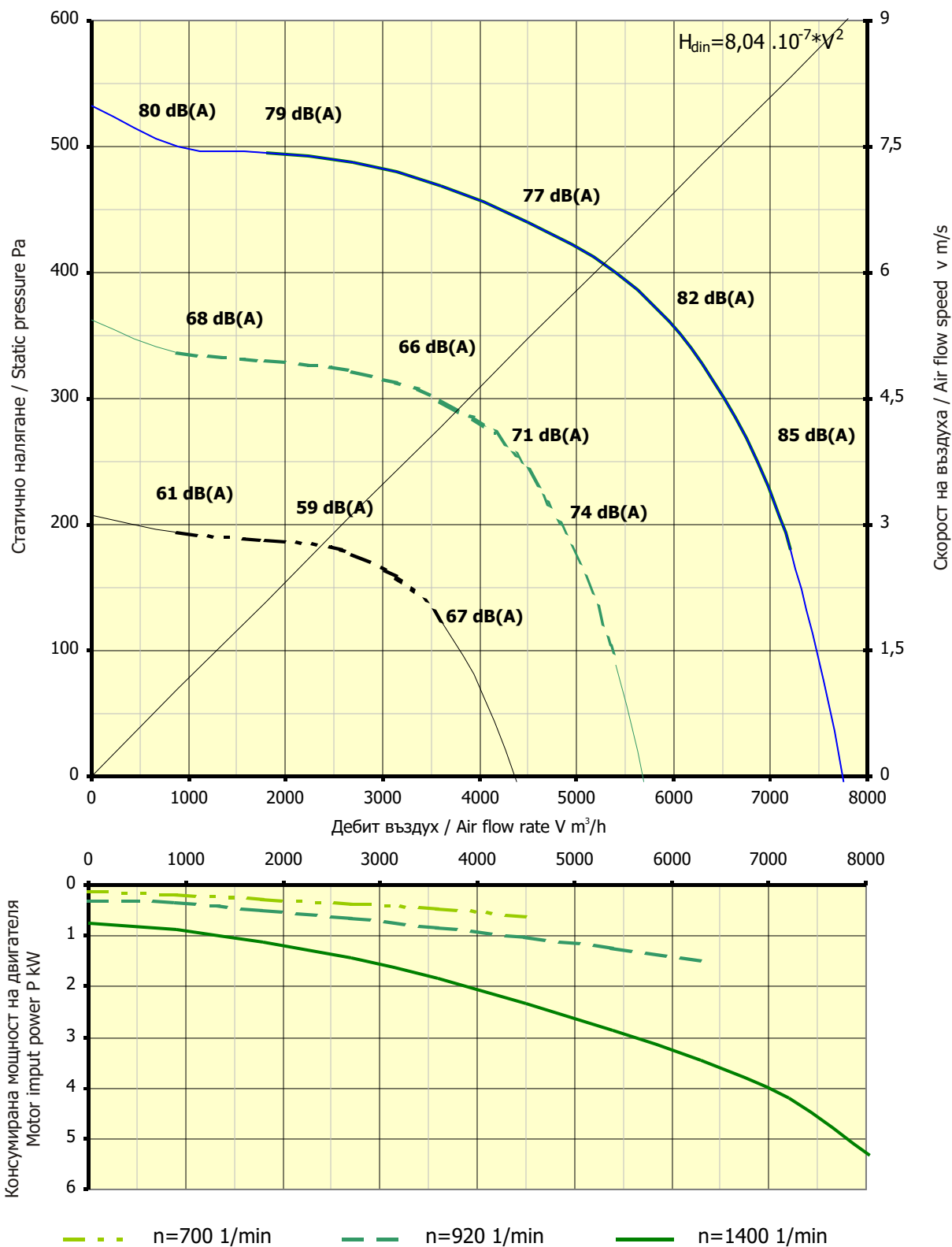
Характеристики на центробежен вентилатор Characteristics of centrifugal fans range KVB-315-600/400 A1
