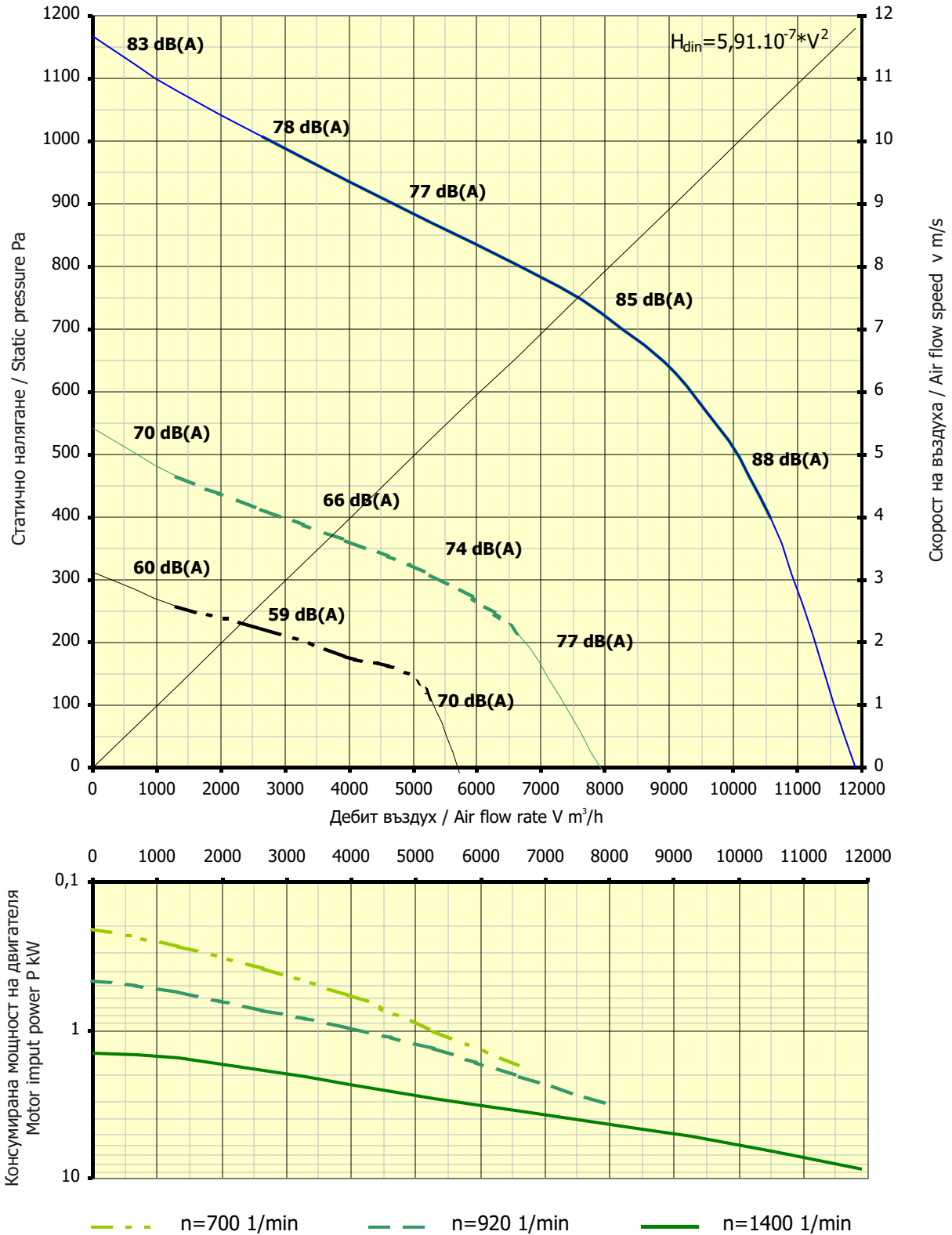
Характеристики на центробежен вентилатор Characteristics of centrifugal fans range KVB-355-700/400 A1
