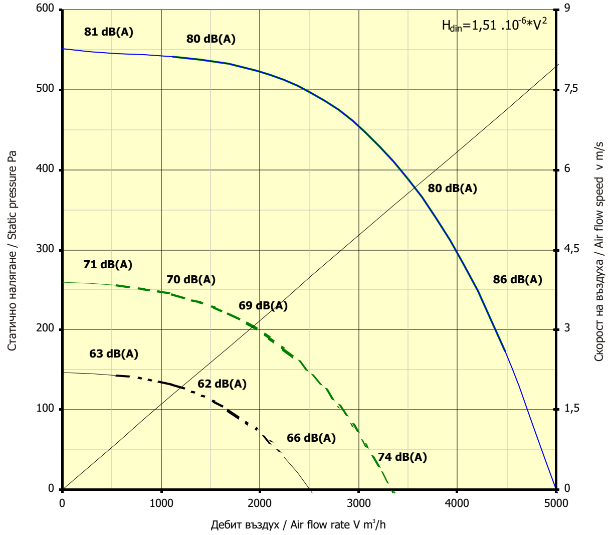
Характеристики на центробежен вентилатор Characteristics of centrifugal fans range KVB-280-500/350 A1
