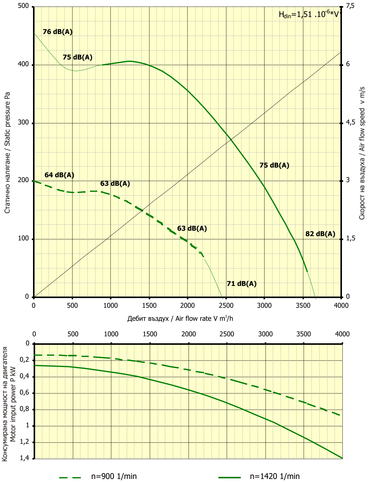
Характеристики на центробежен вентилатор Characteristics of centrifugal fans range KVB-250-500/350 A3
