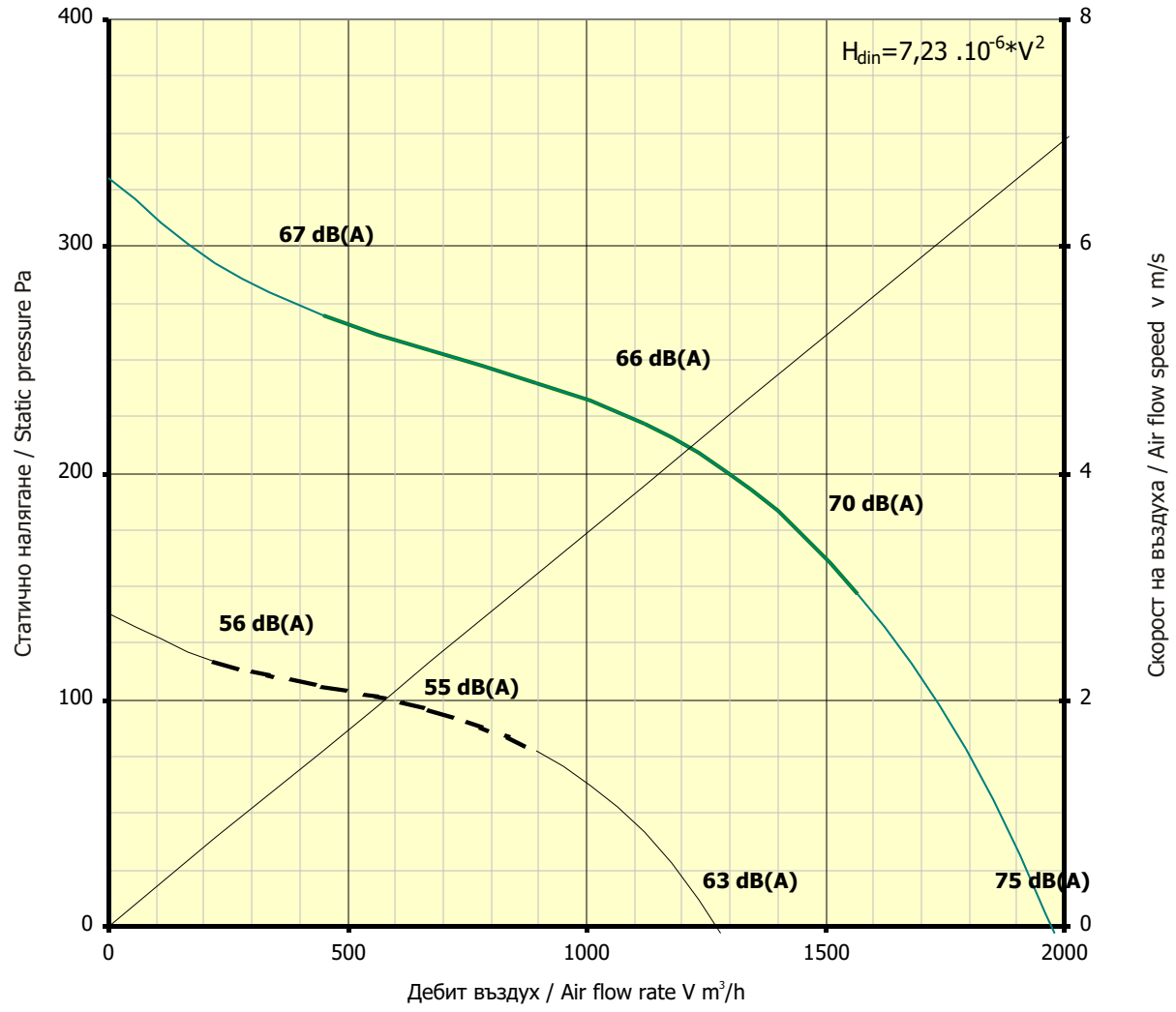
Характеристики на центробежен вентилатор Characteristics of centrifugal fans range KVB-200-400/200 A1
